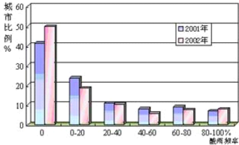
不同酸雨频率城市百分比
