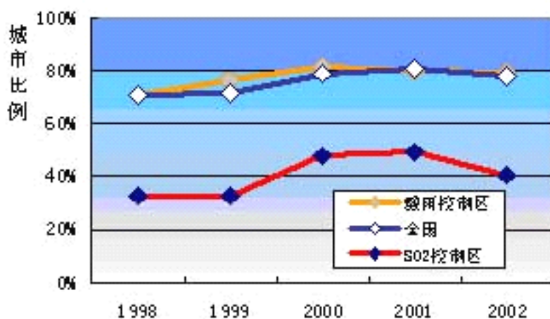
“两控区”SO 2 达标情况
