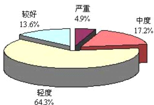
城市道路交通噪声污染程度
