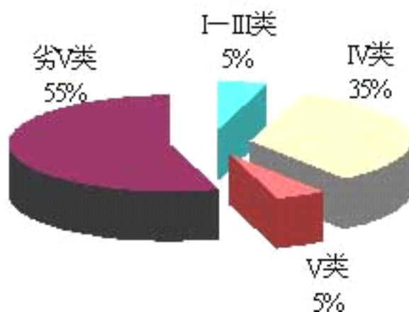
太湖湖体水质类别比例
