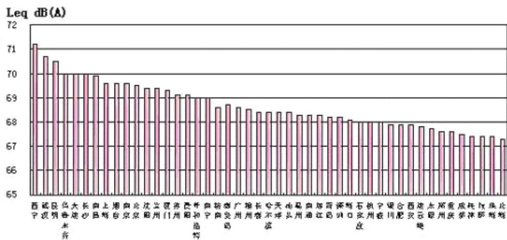
2002年度环保重点城市道路交通噪声等效声级比较
